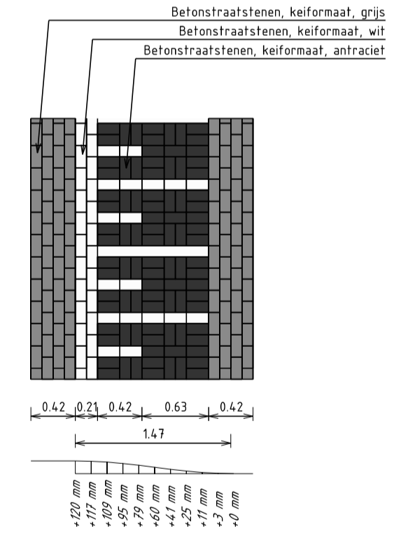
Detail 1: plateau opgang BSS Schaal 1:50
