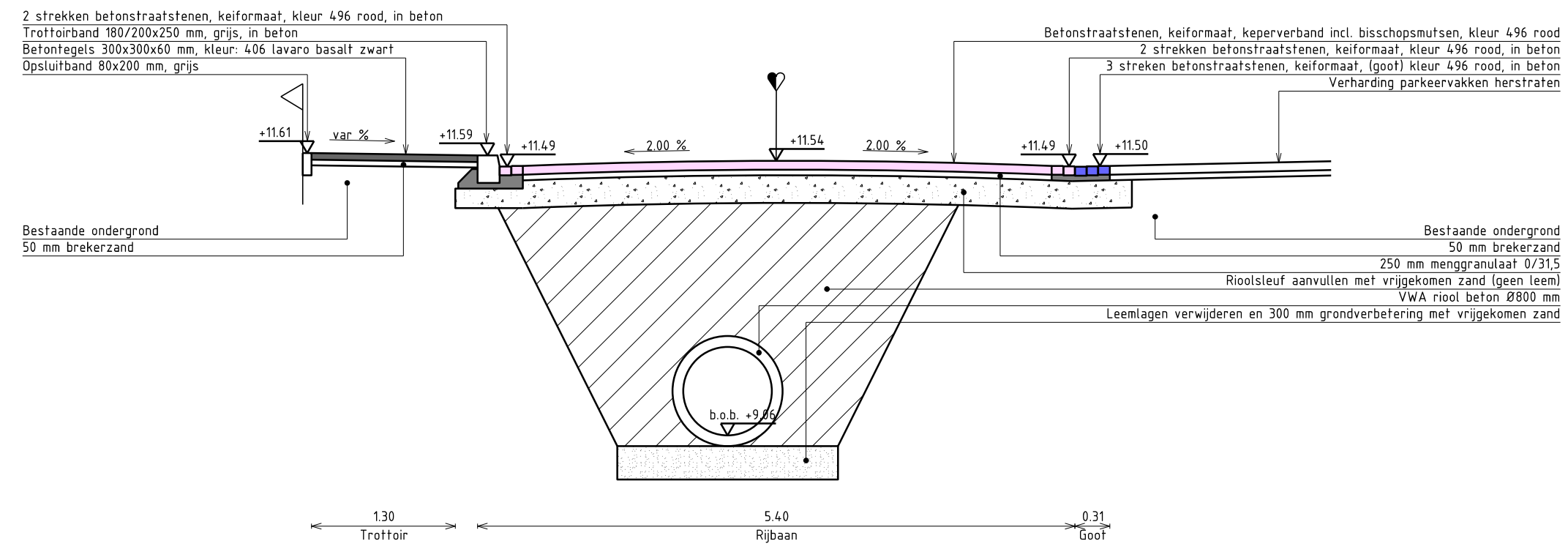
Principe doorsnede A-A Schaal 1:50
